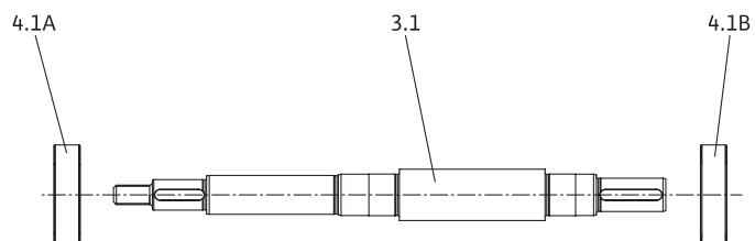
Рис. 23. Опора подшипника
