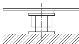
Рис. 7. Нивелирные винты на поверхности фундамента
