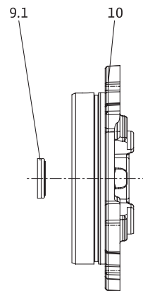
Рис. 27. Крышка корпуса, торцевое уплотнение
