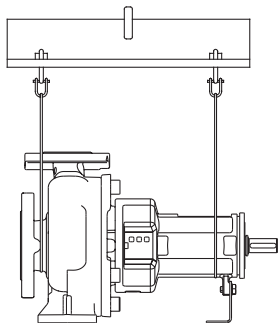
Рис. 3. Строповка насоса
