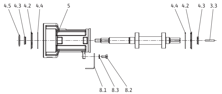
Рис. 26. Опора подшипника
