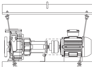
Рис. 4: Строповка агрегата
