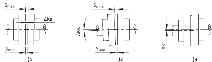
Рис. 11. Выверка муфты без проставки
