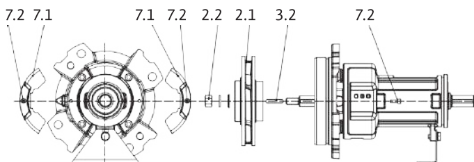
Fig. 20. Демонтаж вставного блока
