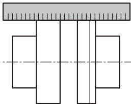
Рис. 14. Проверка радиальной выверки при помощи линейки
