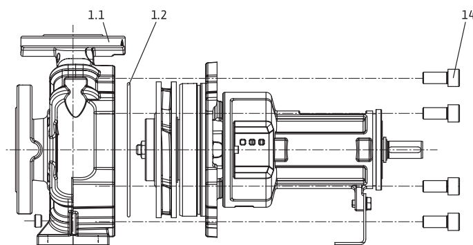
Рис. 30. Установка вставного блока
