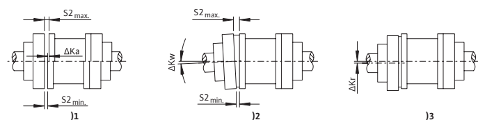
Рис. 12: Выверка муфты с проставкой
