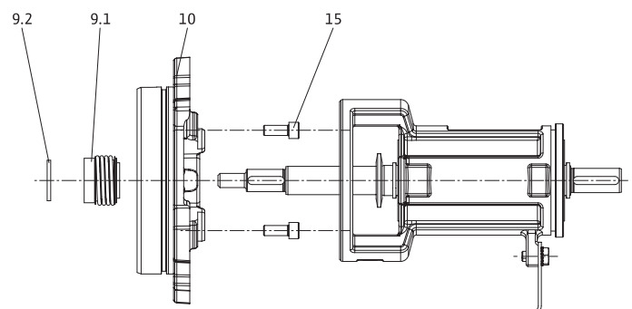
Рис. 28. Исполнение с торцевым уплотнением
