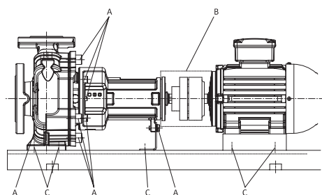
Рис. 31. Крутящие моменты затяжки винтов
