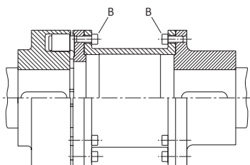
Рис. 18. Винты В крепления полумуфт
